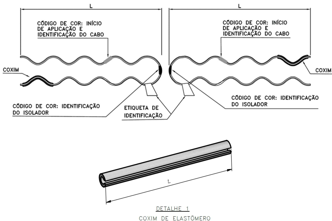
Figura 6 - Laço lateral duplo para condutores de alumínio nus
