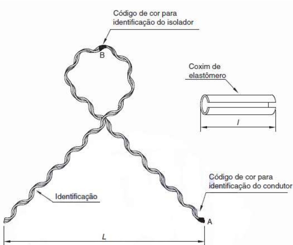
Figura 8 - Laço de roldana para condutores de alumínio
